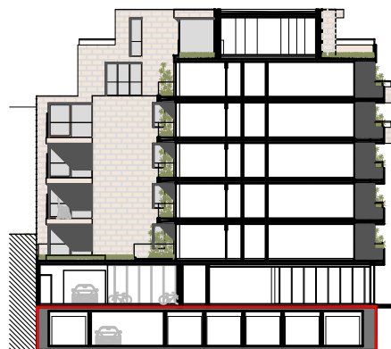
ACHTERGEVEL TOEKOMSTSTRAAT
